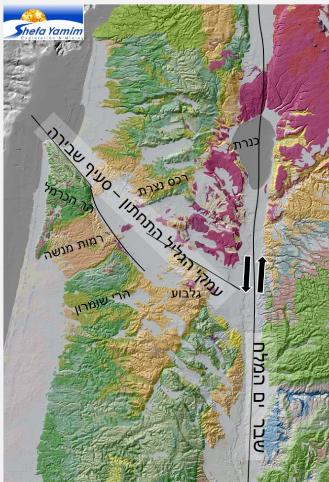
מפה גיאולוגית של צפון ישראל (1:200,000 סנה וחבריו 1998): שבר ים המלח וסעיפו לצפון מערב. עמקי הגליל התחתון ושוליהם, הכרמל, רמות מנשה, הרי שומרון, גלבוש, גבעות הגליל המזרחי ורכס נצרת
