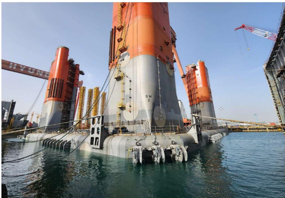
חלקו הצף של ה-FPS (Hull) במתקני מספנת HHI
